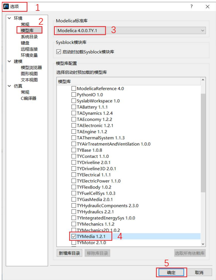
图 2-10 模型库加载（方式二）
